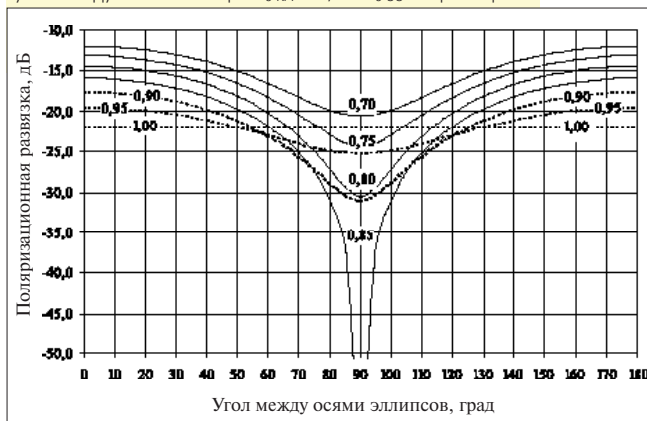
Рис. 2. Зависимость уровня поляризационной развязки от угла между эллипсами при K_{\Sigma \text{ КА}} = 0,85 . K_{\Sigma \text{ ЗС}} - параметр
