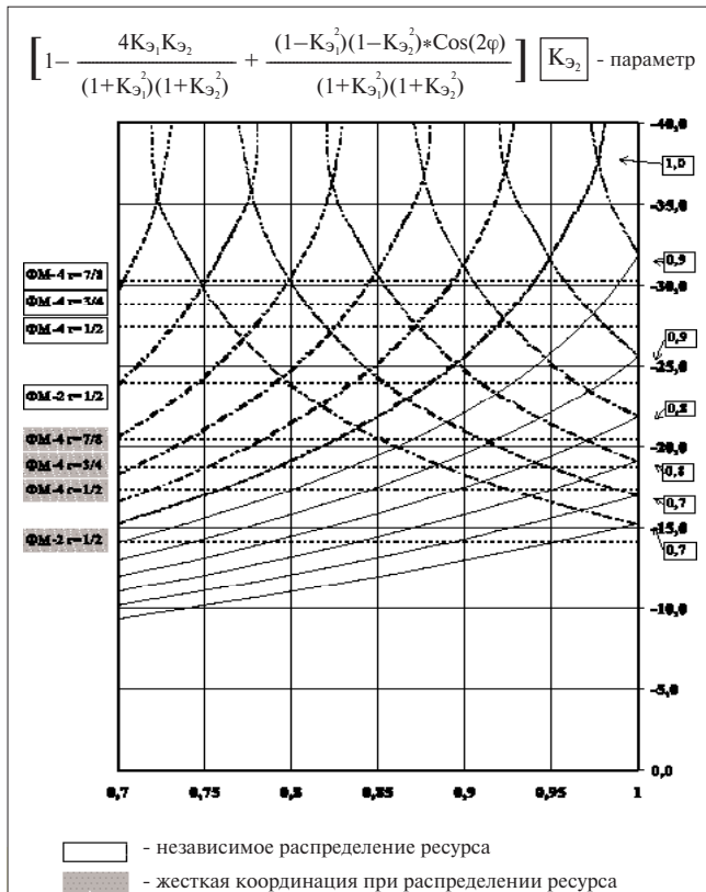
Рис. 1. Поляризационная развязка для разных K_{\Sigma} при соосном ( \varphi=0 ) и ортогональном ( \varphi=\pi/2 ) расположении эллипсов поляризации
